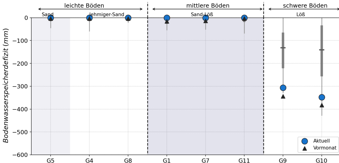
Abbildung 3: Ausschöpfung des Bodenwasserspeichers der Wurzelzonen der untersuchten Lysimetergruppen für Ende Januar 2023 (blauer Kreis) im Vergleich zum Vormonat (Dreieck) und der Beobachtung im Referenzzeitraum 1991 – 2020 (graue Boxplots: unteres Ende – Minimum, graue Box – 25 % und 75 % Perzentil, Strich – Median, oberes Ende – Maximum)
